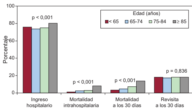
Figura. Resultados evolutivos de los pacientes durante el ingreso y el seguimiento a corto plazo por grupos de edad. Significación calculada mediante prueba de la \chi^2 de tendencia lineal.
