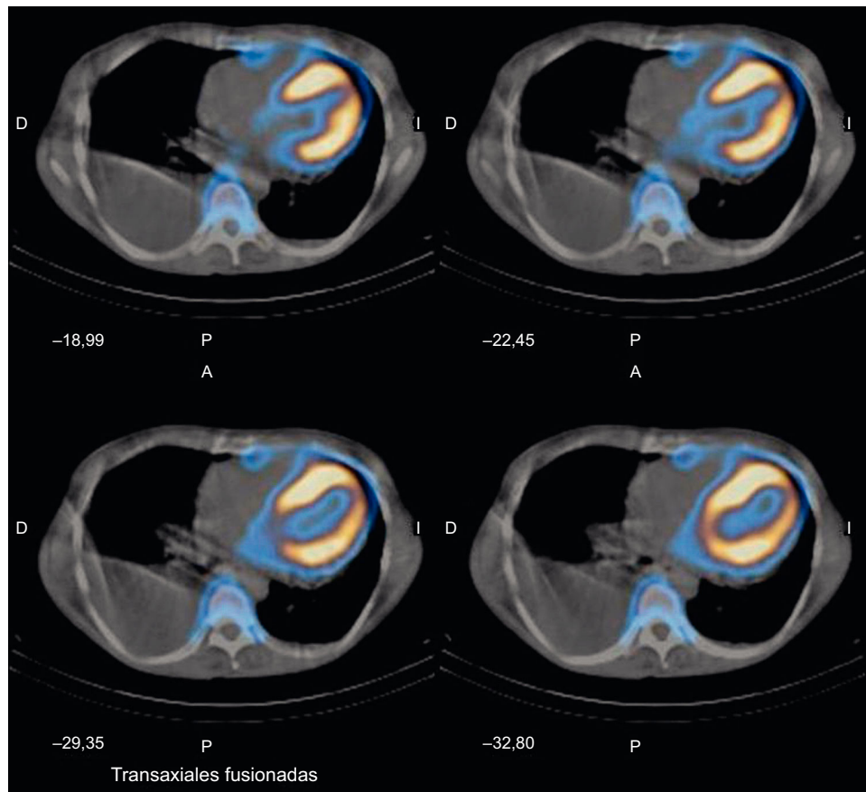
Figura 2. Gammagrafía ósea con ^{99m}\text{Tc} -2,3-dicarbóxipropano-1, 1-difosfonato y tomografía computarizada por emisión monofotónica combinadas con una tomografía computarizada convencional, que muestran un aumento en la cantidad de sangre miocárdica biventricular durante la fase inicial, además de una intensa captación de radiotrazador en ambos ventrículos durante la fase tardía. A: anterior; D: derecho; I: izquierdo; P: posteroanterior.
